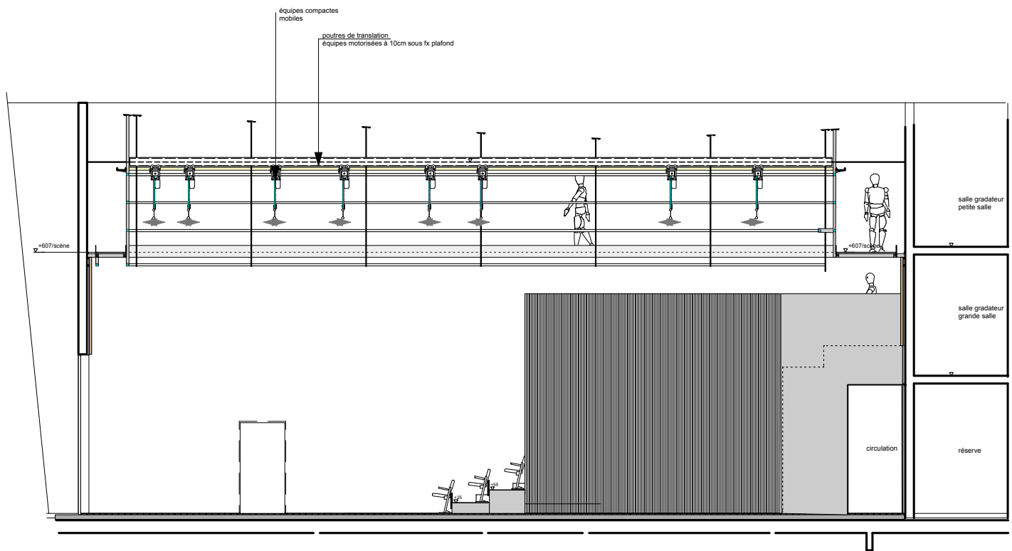
COUPE SC Longitudinale CC'
