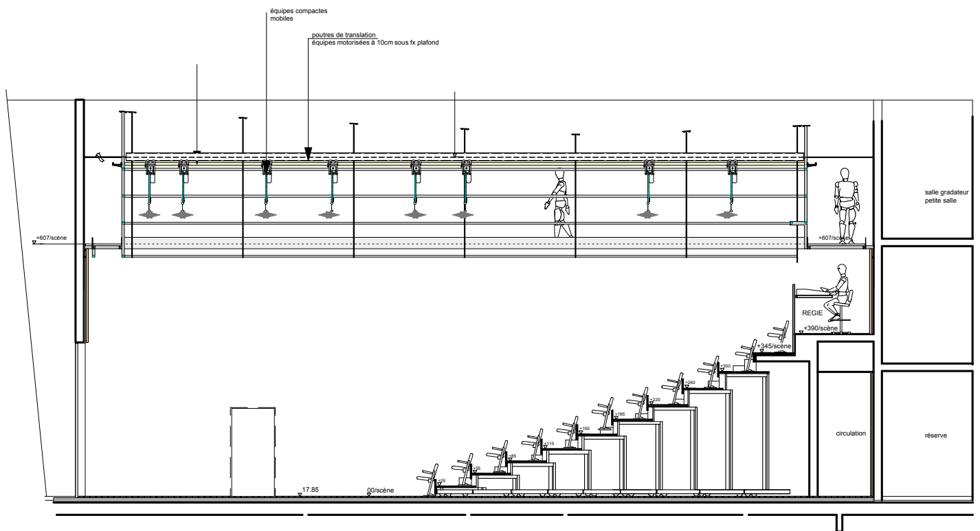
COUPE SC Longitudinale axe scène
